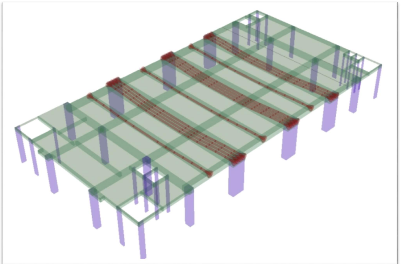
Mặt bằng cáp dầm sàn tầng 2 – Khẩu độ 28m
